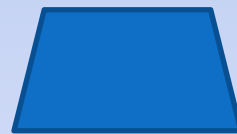
quadrilaterals
