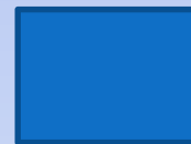
quadrilaterals
